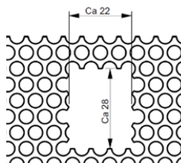
Udsnit i gitteret på kølebaffel.
